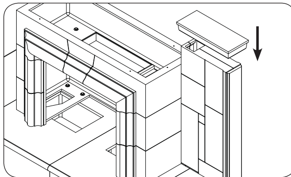
Fig. 18-5 Assemble top side-wall (skip if n/a)
