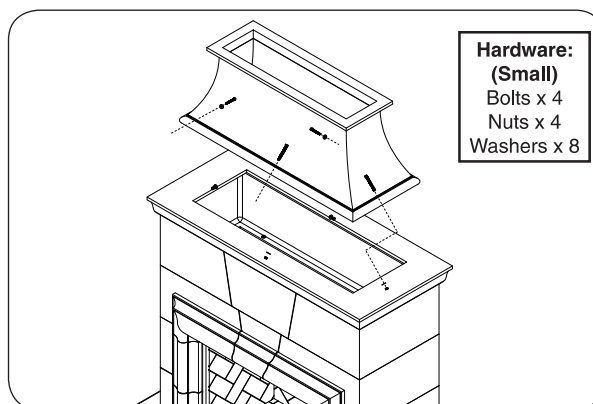
Fig. 19-3 Assemble chimney
