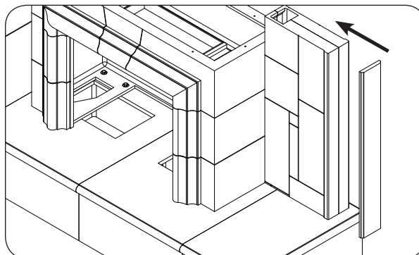
Fig. 18-4 Assemble end side-wall (skip if n/a)
