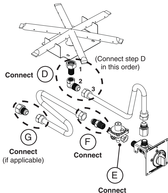
Fig. 3-2 New configuration (Nat. gas)
