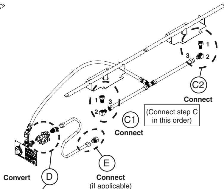
Fig. 11-2 New configuration (Nat. gas)
