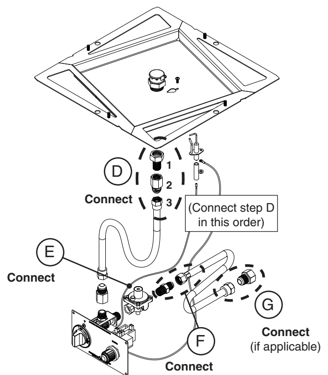
Fig. 7-2 New configuration (Nat. gas)
