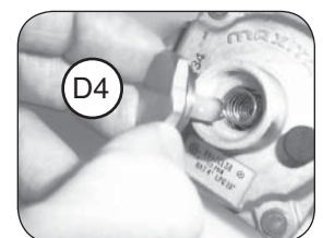
Fig. 5-2 New configuration (Nat. gas)
