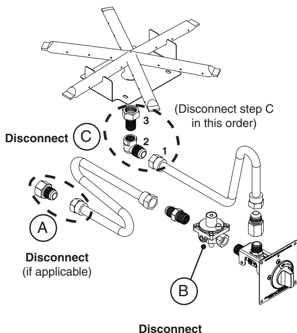
Fig. 4-1 Original configuration (Nat. gas)
