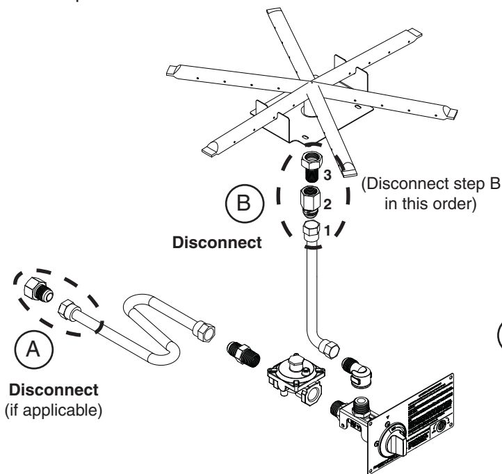
Fig. 6-1 Original configuration (Nat. gas)
