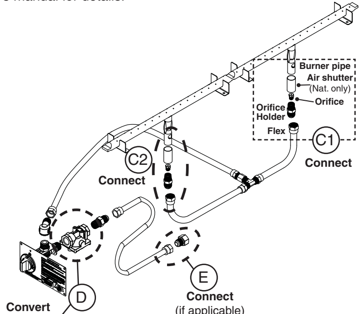
Fig. 13-2 New configuration (Nat. gas)
