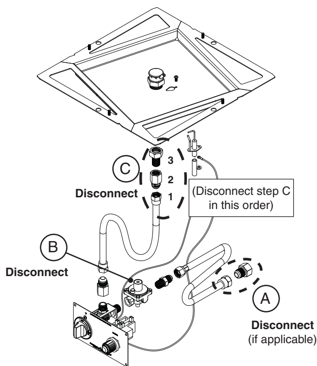
Fig. 8-1 Original configuration (Nat. gas)
