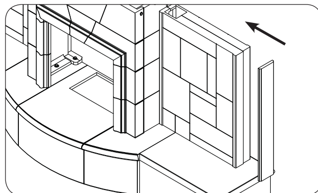
Fig. 20-3 Assemble end side-wall (skip if n/a)
