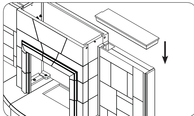
Fig. 20-4 Assemble top side-wall (skip if n/a)
